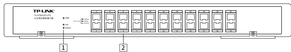
图1-21 TL-ST8022F-LPU结构示意图
